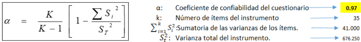
Fig. 1. Alfa de Cronbach
